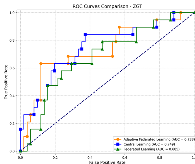
FIGURE 5 ROC curve comparison for the test center ZGT. ZGT, Ziekenhuisgroep Twente.
